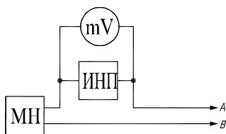
Рисунок Б.9 - Схема проверки влияния помехи нормального вида
