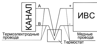
Рисунок Б.2 - Схема подключения входного сигнала от термопары с термокомпенсацией
