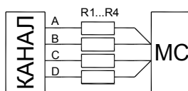
Рисунок Б.4 - Схема подключения входного сигнала от термопреобразователя сопротивления по 4-х проводной линии связи
