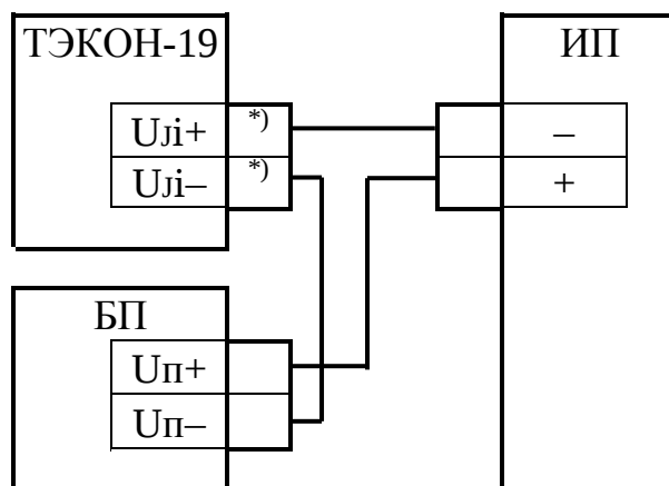
б) двухпроводная
